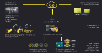
ОБЩАЯ СХЕМА КОМПЛЕКСА
